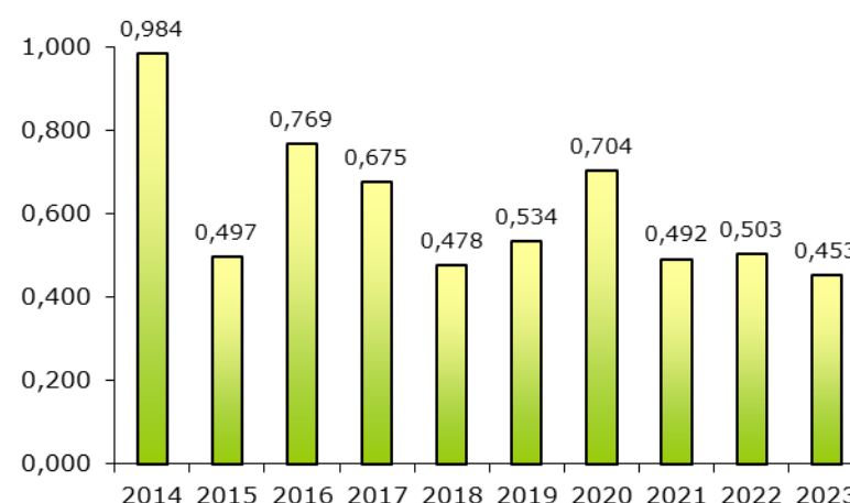
Consumo de pellets (MWh/trabajador)
